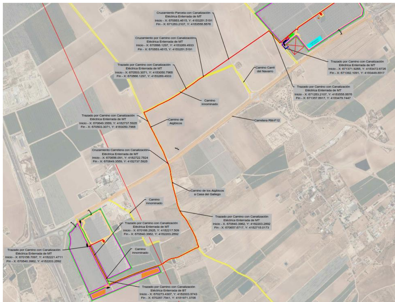
Figura 1: Cruzamientos Canalizaciones Elec. Con Caminos Públicos
